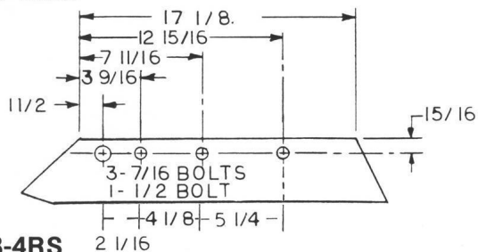
IH16-4RS IH16-4LRS
